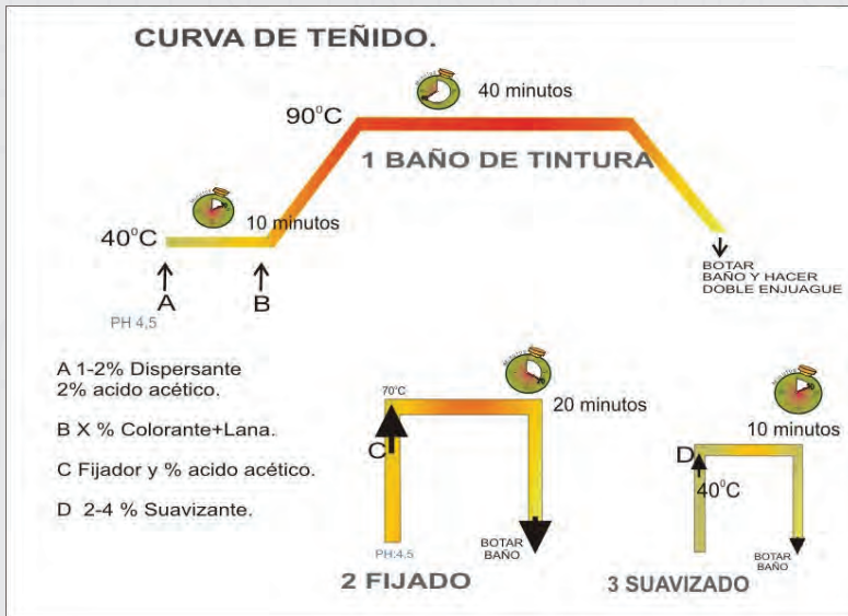
CURVA DE TEÑIDO, PROPUESTA Fuente: Carol Valencia C. 2007
