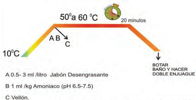
CURVA LAVADO DE VELLÓN PROPUESTA Fuente: Carol Valencia C.2007
